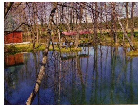
На выходе подземные воды образуют небольшой озеровидный водоем
